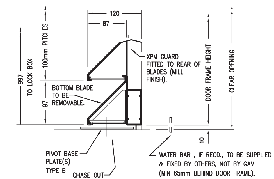
721. DOOR CILL
