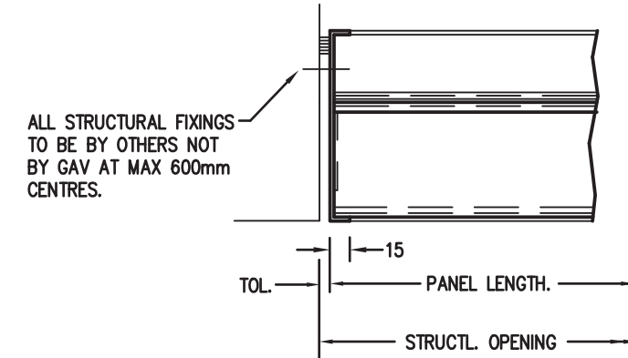
709. JAMB DETAIL
