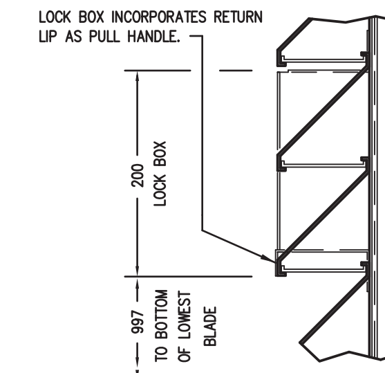
722. LOCKBOX
